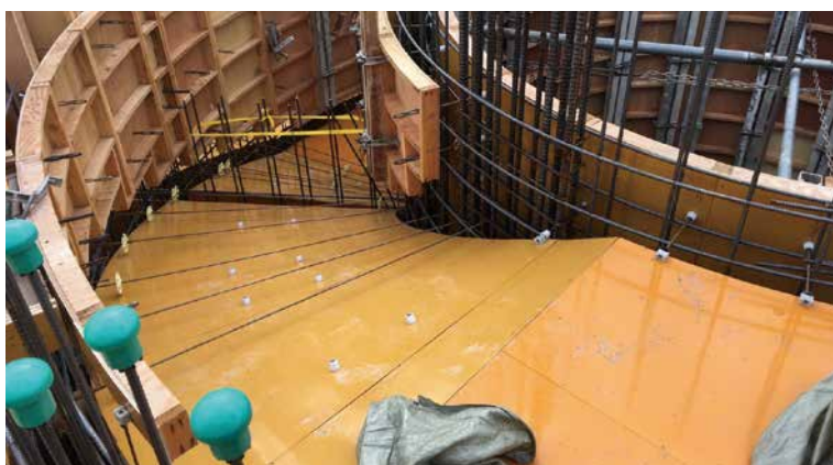
らせん階段
