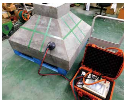
透気係数測定状況
