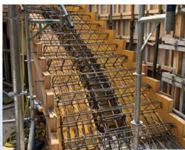
らせん階段
