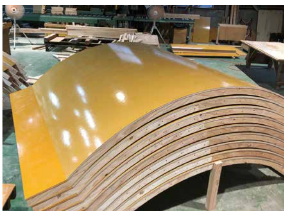
波返し型枠
