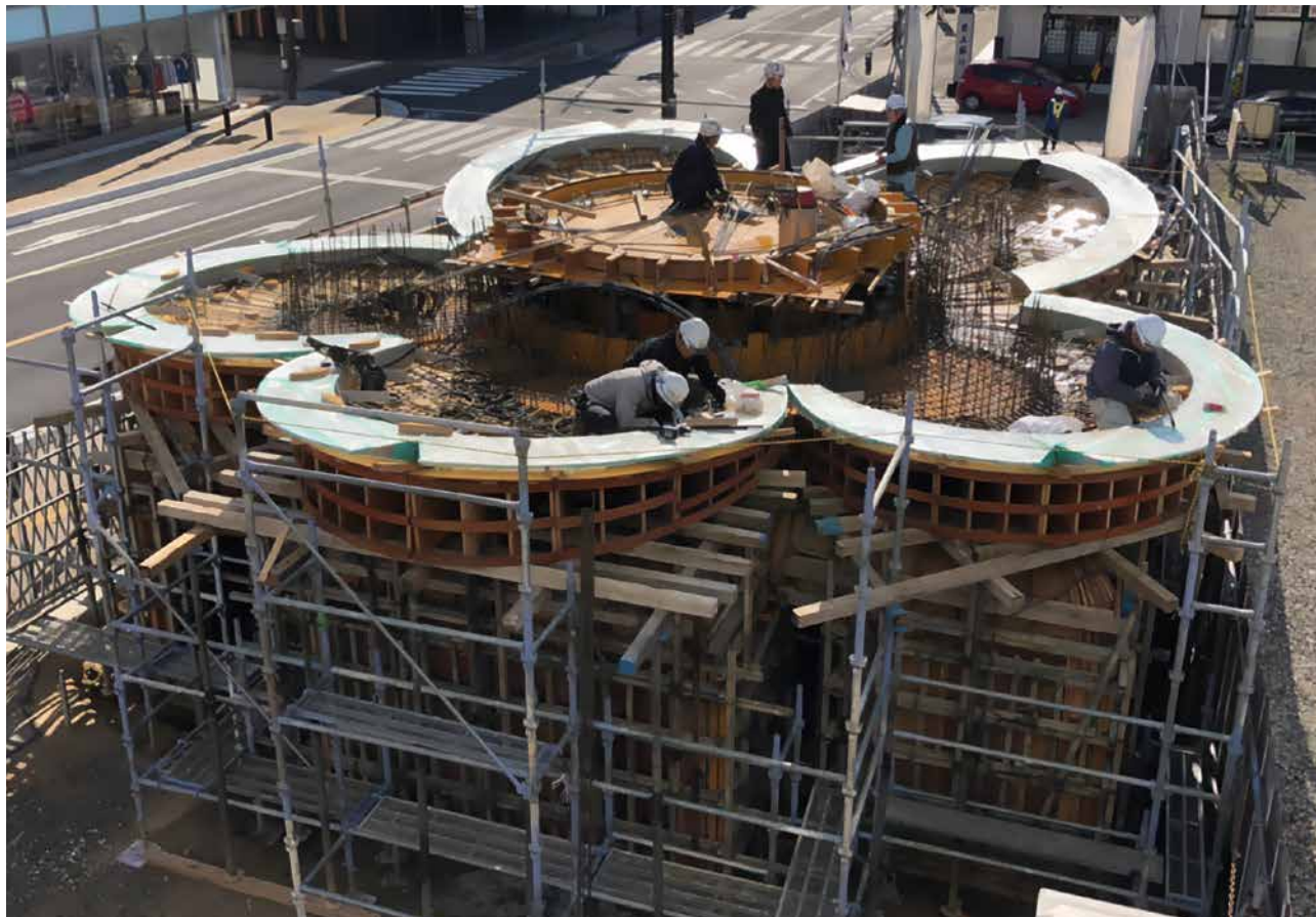
特殊スラブ底型枠
