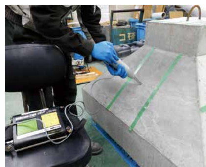
反発度測定状況
