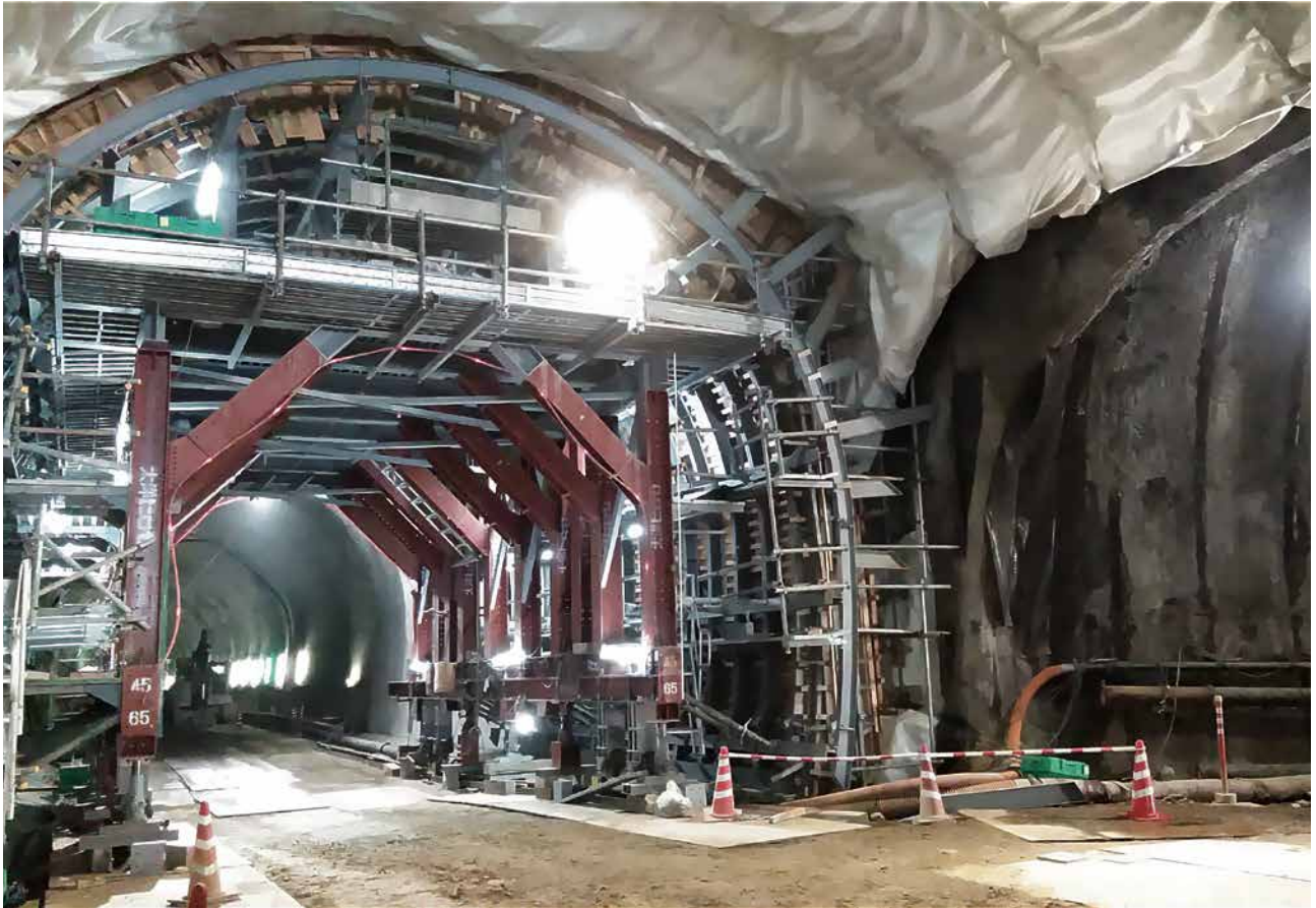
トンネル交差部パラセントル
