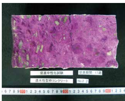
促進中性化試験（アクアトール）
